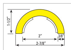
Type R2: 39-3/8" x 2-7/8" x 1-1/2"
